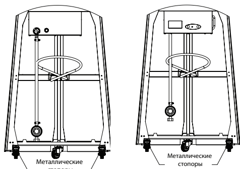
Рис.9 - Установка стопоров
