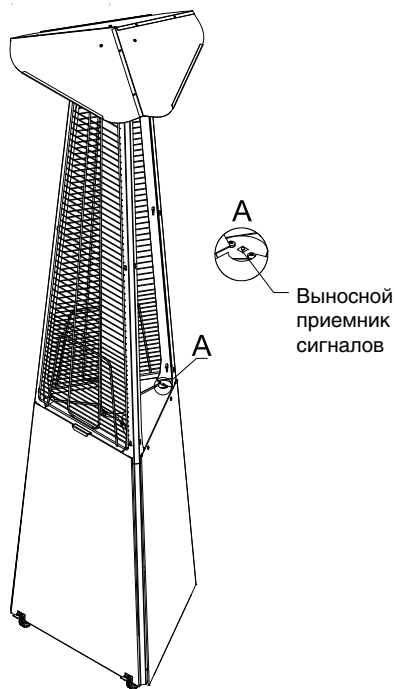
Рис.8 - Положение датчика модели BOGH-15E
