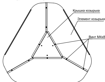
Рис.15 - Сборка козырька
