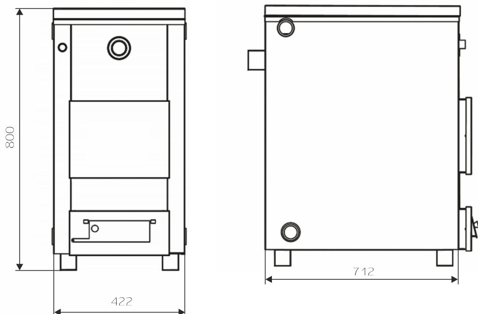
Рис. 3 Габаритные размеры котла «Сибирь-Гефест» 20 кВт
